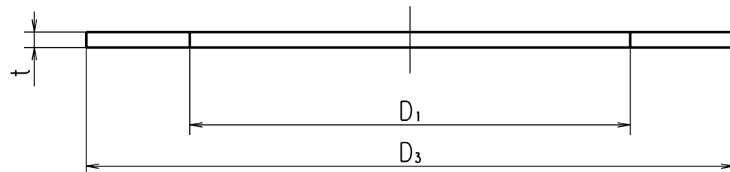
RF形ガスケット
