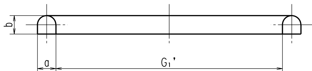
GF形ガスケット 1号
